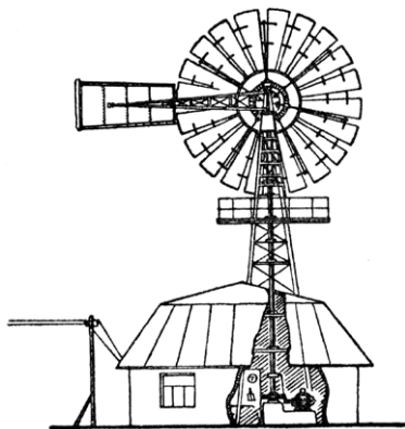
Рис. 47. Ветряной двигатель.
